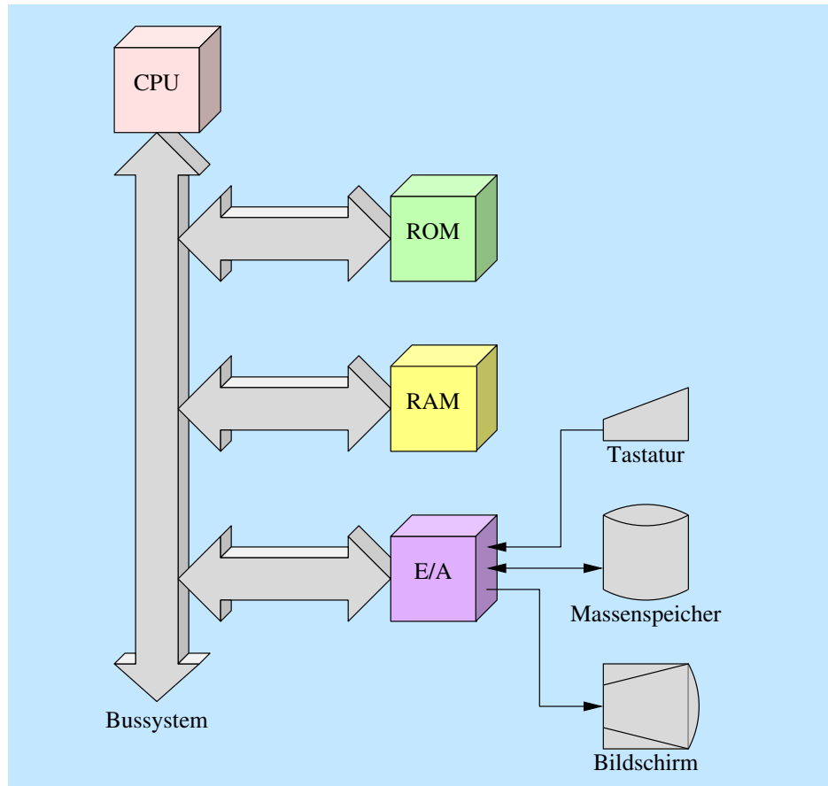
Abbildung 1: Bus-Topologie, logisch
